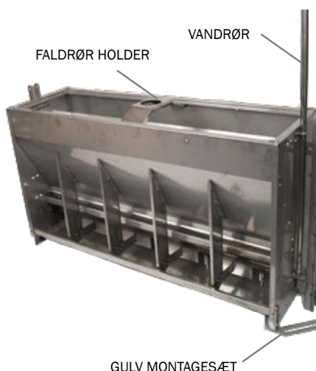
GULV MONTAGESÆT
