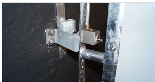
Vinkel beslaget monteres og virker som bagstop
