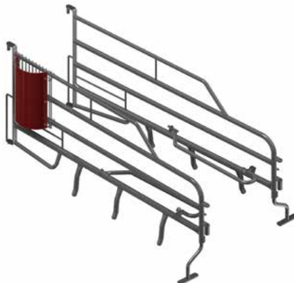
Halmhæk på farelad XL. Kan placeres i begge sider.
