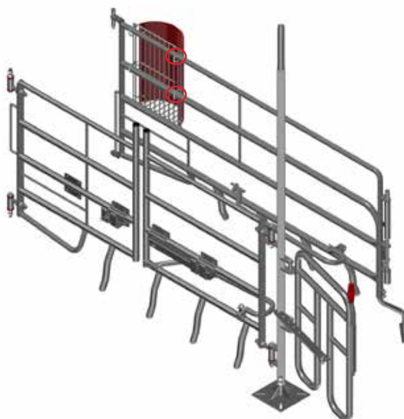
Halmhæk på farelad, Farrow Comfort. Monteres på første og anden rør i skillerummet. Har også mulighed for montering på andet og fjerde rør. Monteres på en fuld væg uden åbninger
