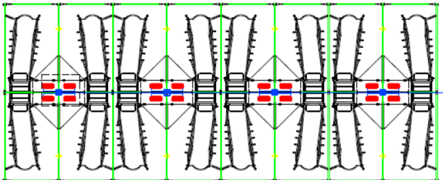
Installation af 16 Master Heater med 8 Dobbelt kontakter
