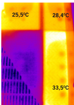
Termografisk varmfordeling for plastvarmeplade
